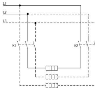
400 V cables
