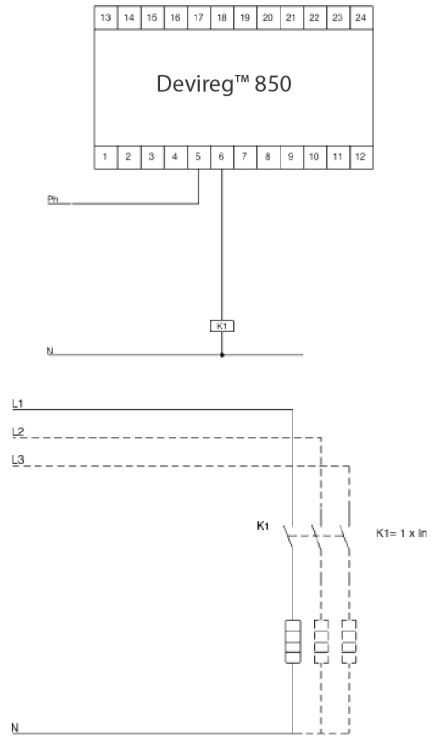
230 V cables
