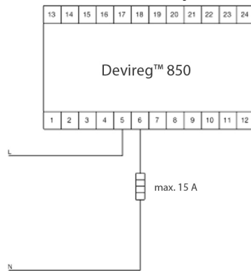
230 V cables
