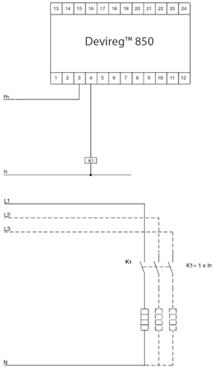
230 V cables
