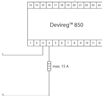
230 V cables
