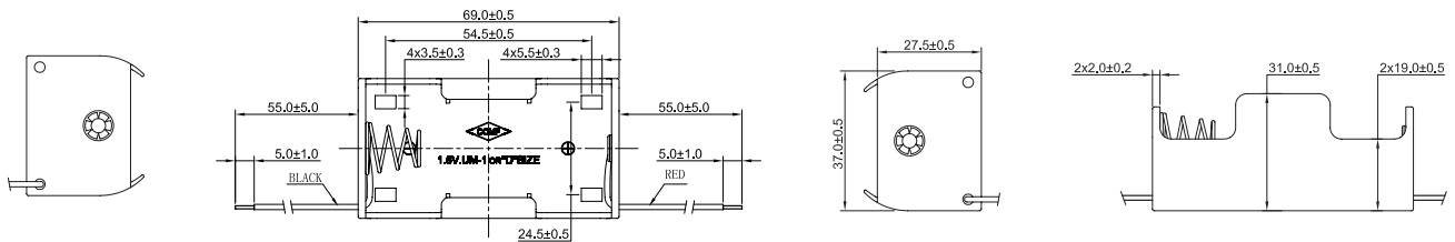
Dimensions : Millimetres
