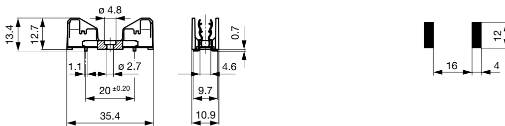
Anschlussflächen
