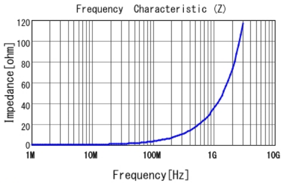
■ LQW18AN5N6G80 |Z|
