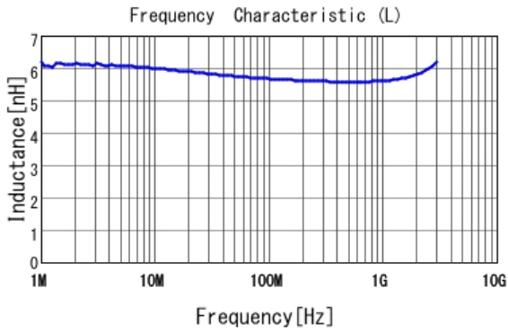
■ LQW18AN5N6G80 L
