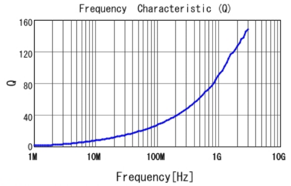
■ LQW18AN5N6G80 Q
