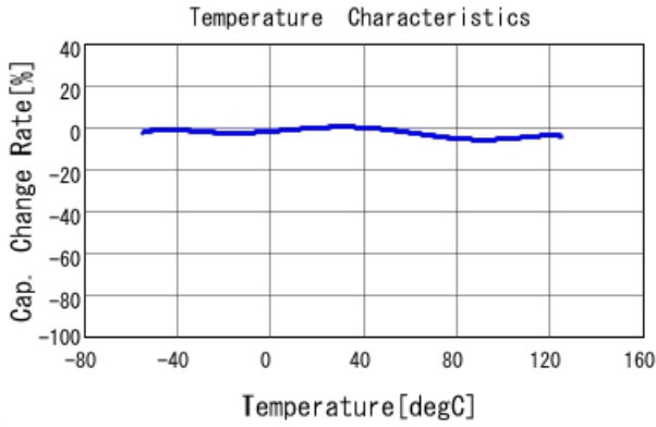
■ GCJ21BR72A104KA01 C-Temp. capchange, DCO. 0V, AC1. 0Vrm
