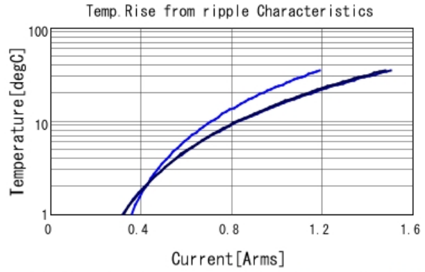
GCJ21BR72A104KA01 Temp. rise ■ 400kHz ■ 800kHz ■ 1MHz
