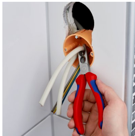
Ściąganie izolacji z przewodów w puszkach instalacyjnych
