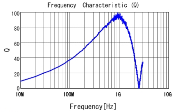
■ LQW2BAS39NG00 Q
