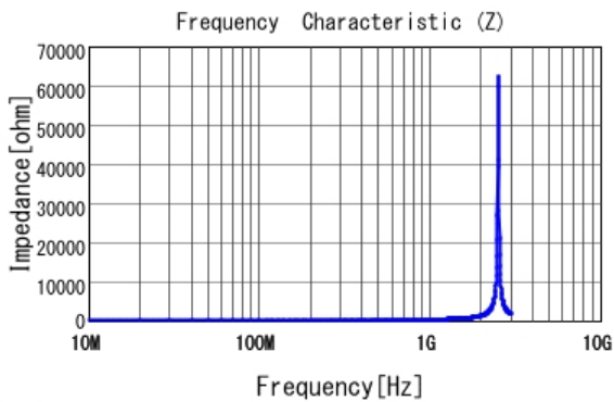
■ LQW2BAS39NG00 |Z|
