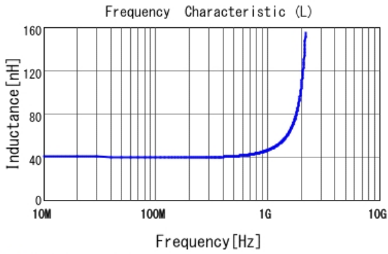
■ LQW2BAS39NG00 L
