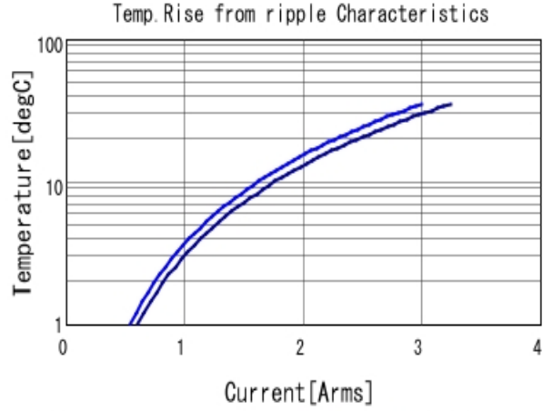
GRM033R60J225ME15 Temp. rise ■ 500kHz ■ 1MHz
