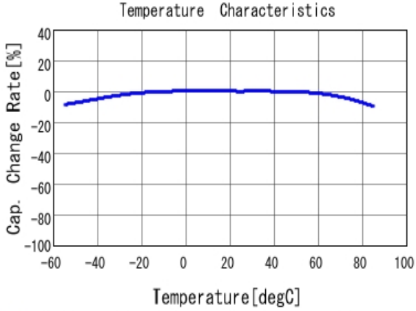
■ GRM033R60J225ME15 C-Temp. capchange, DCO. 0V, ACO. 1V rm
