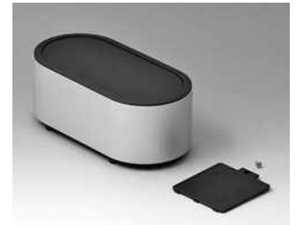
EO186059 SYNERGY O180 Aluminium AlMgSi 0,5 matt eloxiert 180x90x70mm IP 40
