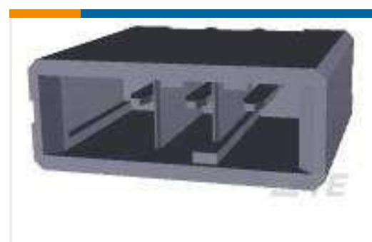
TE Teilenummer2-178136-3 DYNAMIC D3200 HDR V ASSY 3P
