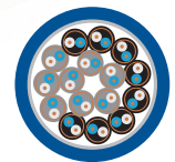
Schnittzeichnung
