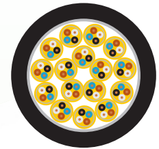
Schnittzeichnung
