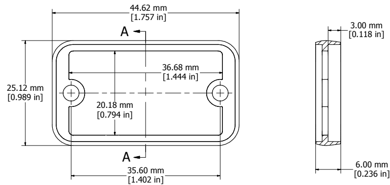
OPEN BEZEL
