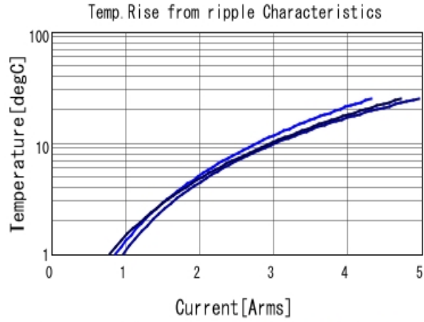
KRM55WR72A156MH01 Temp. rise ■ 50kHz ■ 100kHz ■ 300kHz
