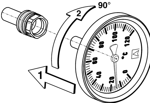
Bild 3: Montage
