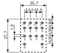
Ansicht auf die Anschlüsse
