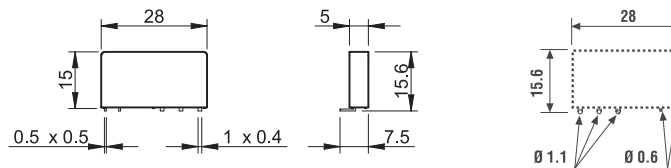
Ansicht auf die Anschlüsse
