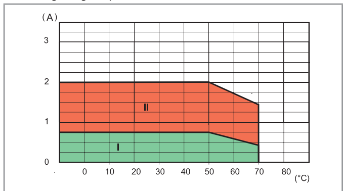
L 34 - Ausgangsbelastbarkeit - Dauerstrom in Abhängigkeit von der Umgebungstemperatur, 34.81.7...8240
