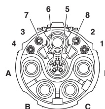
Polbild Buchse Signal, Kodierung 1
