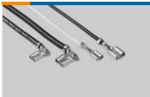
Schnelltrennanschlüsse(4)
