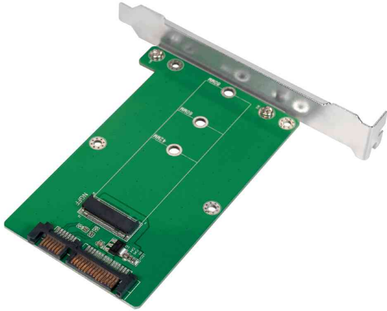
SATA - M.2 SATA SSD Schnittstellenkarte
