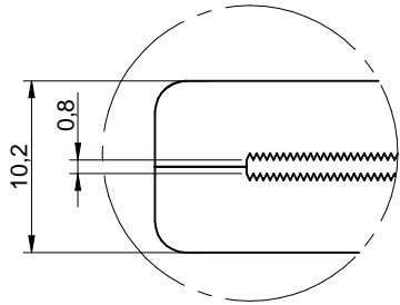
2:1 detail A
