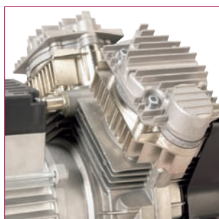
Zweizylinder-Kompressor mit großen Kühlflächen
