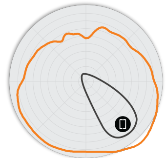
Abbildung 5. R650 5 GHz-Elevation-Antennenmuster
