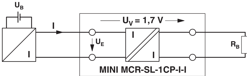
Applikationszeichnung
