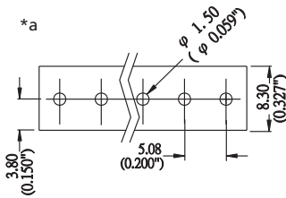
*a Leiterplattenlayout
