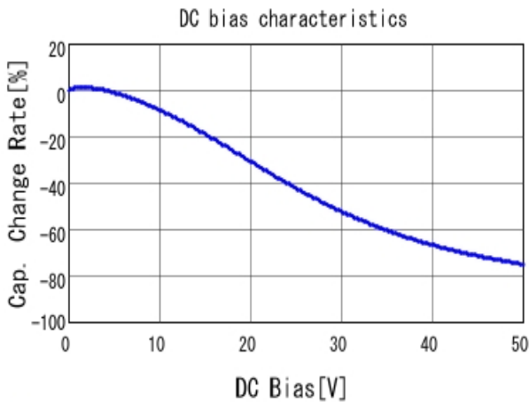
■ GCJ31CC71H475KA01 C-DC bias capchange, 25.0degC, AC1.
