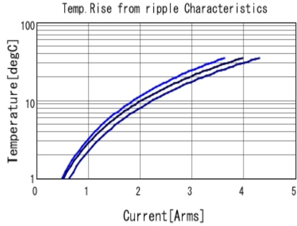
GCJ31CC71H475KA01 Temp. rise ■ 100kHz ■ 500kHz ■ 1MHz
