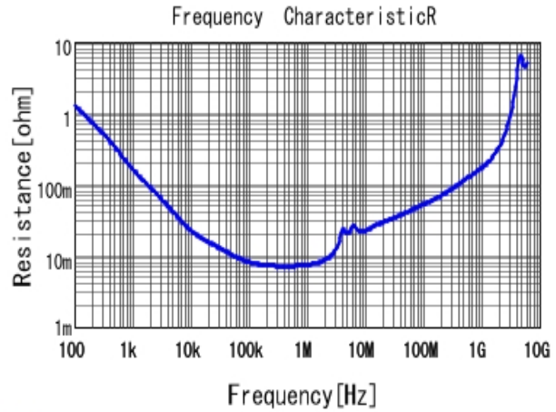
■ GCJ31CC71H475KA01 R DC0V, 25degC
