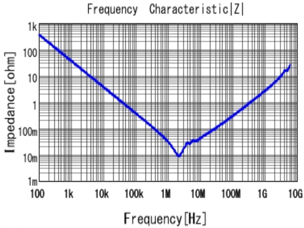
■ GCJ31CC71H475KA01 |Z| DC0V, 25degC
