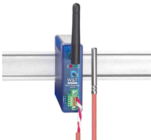
Visuel de référence : thermomètre WiFi 1 x Pt100
