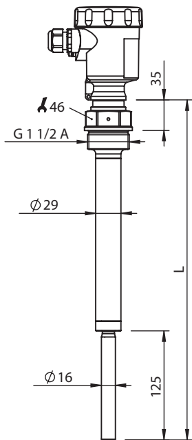
LBV331 Gewindeausführung G 1 1/2 A
