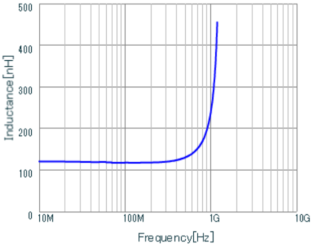
LQP03HQR12J02 L.
