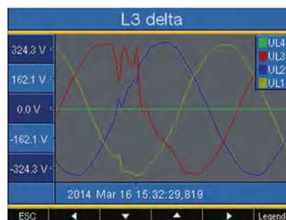
Abb.: Graphische Darstellung einer Transiente
