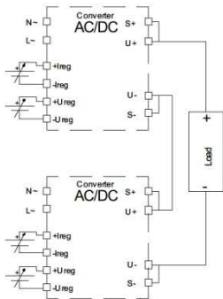
Serienschaltung (Fig.1)
