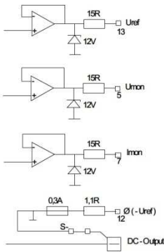
Monitor Ausgänge Schema (Fig.1)
