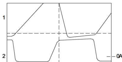
Dynamische Lastreaktion ohne Stromsenke: negativer Laststrom durch Rückspeisung entsteht
