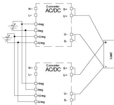
Parallelschaltung (Fig.2)
