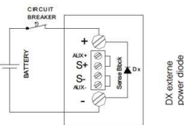
Batterielader-Modus (Fig.7)
