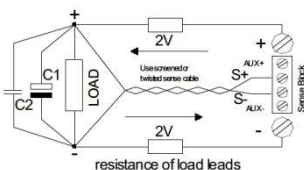
Maximal mögliche Kompensation (Fig.9)
