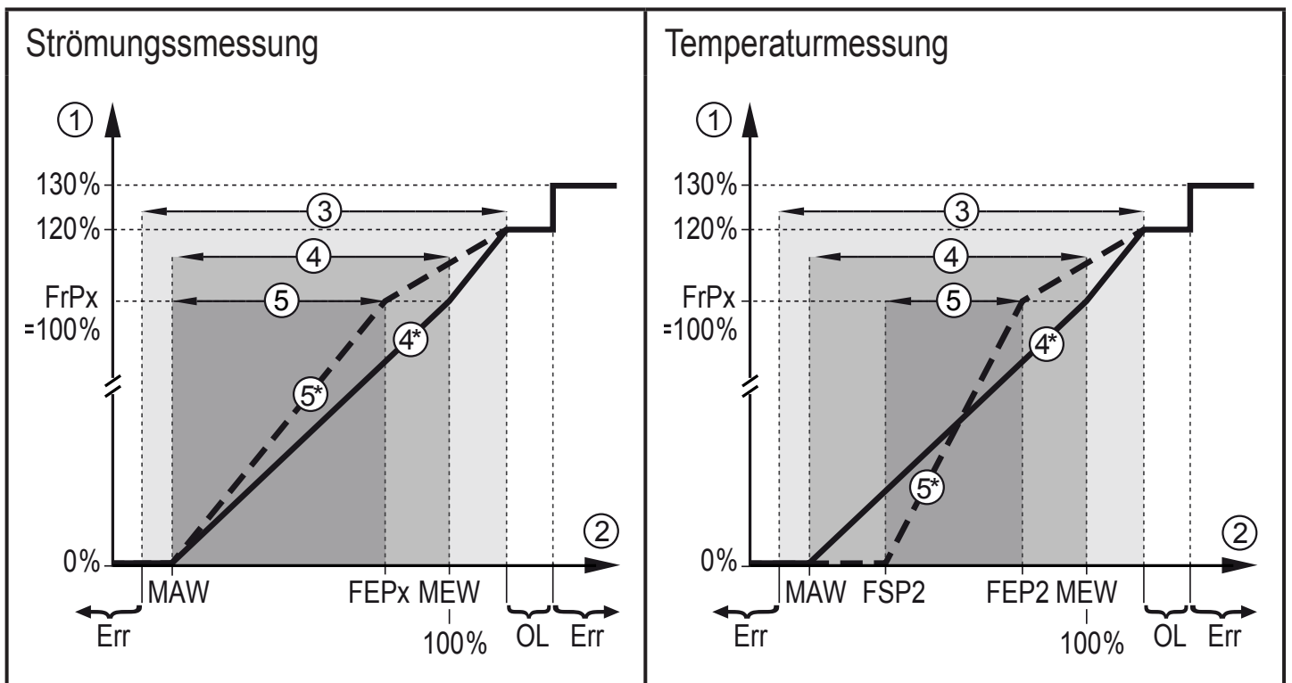
Abbildung 1: Ausgangskennlinie Frequenzausgang
