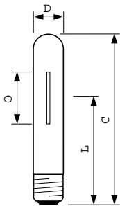
MASTER SON-T PIA Plus 70W/220 E27 1SL/12
