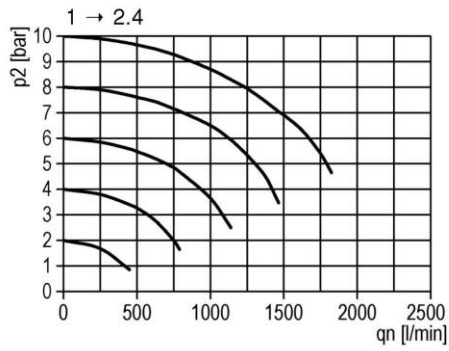
2. Durchflussdiagramm
