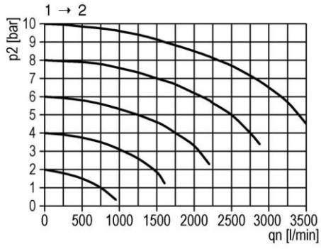
1. Durchflussdiagramm
