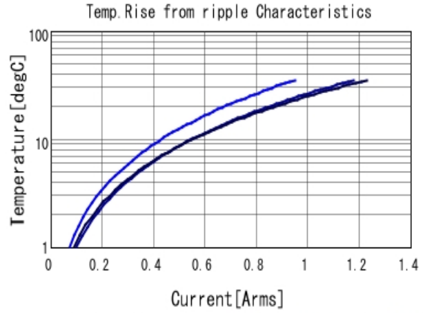
GCM155R71C154KE02 Temp. rise ■ 400kHz ■ 800kHz ■ 1MHz
