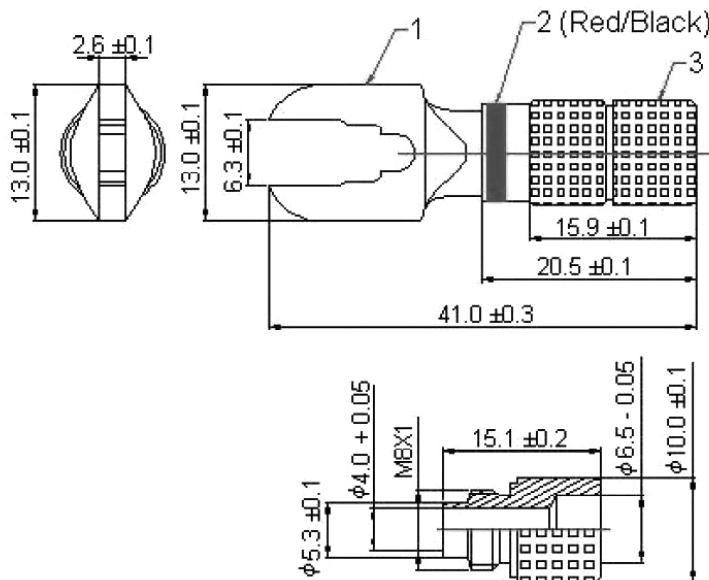
Dimensions : Millimetres
