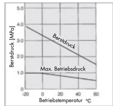
Berstdruckkurve und Betriebsdruckkurve
