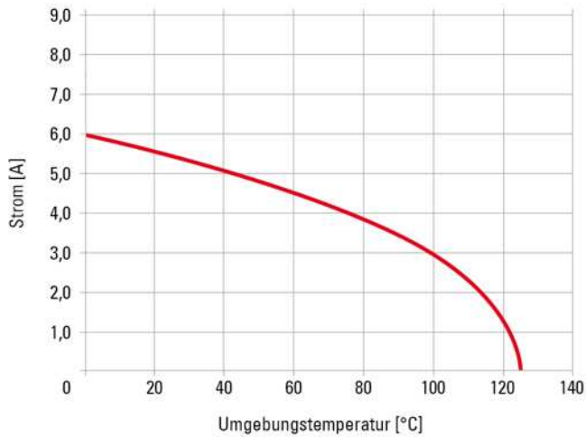
Stromtragfähigkeit Signalkontakte max. 5.5A bei 20°C (2 von 80 polig)
