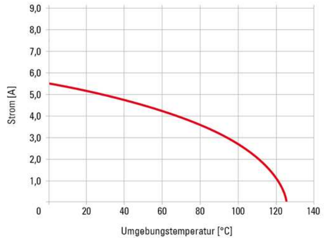
Stromtragfähigkeit Signalkontakte max. 5.1A bei 20°C (4 von 80 polig)
