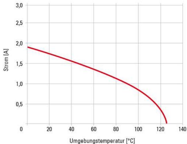
Stromtragfähigkeit Signalkontakte max. 1.7A bei 20°C (80 polig)
