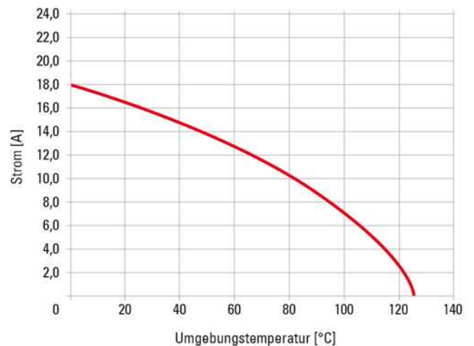
Stromtragfähigkeit Schirm max. 16A at 20°C 80 polig, Bauform mid
