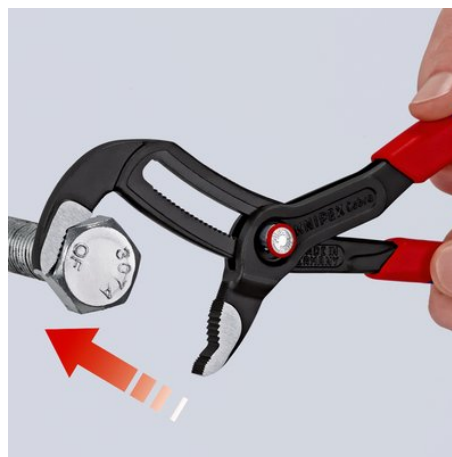
Przyłożyć szczypce i przesunąć szczęki
