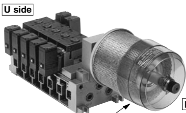
Non plug-in
