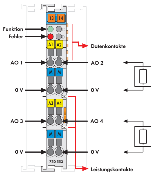
Abb. Serie 750 / Darstellung siehe Seite 24 / Lieferung ohne Mini-WSB Kennzeichnung Serie 750 / 753 siehe Seite 10 ... 11 / 12 ... 13
