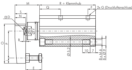
Kolben Ø 20 & 25 mm
