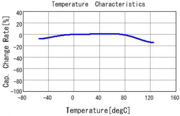
■ GRM32ER71A476KE15 C-Temp. capchange, DCO. 0V, ACO. 5Vrm
