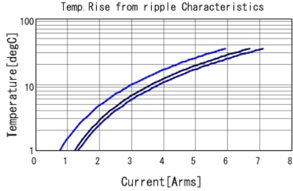
GRM32ER71A476KE15 Temp. rise ■ 60kHz ■ 300kHz ■ 600kHz
