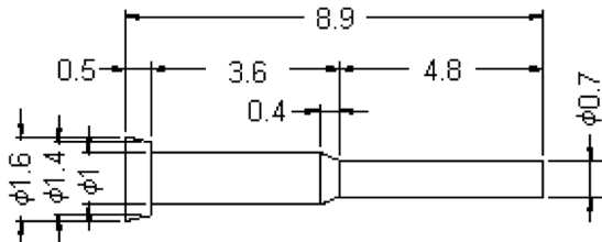
Dimensions : Millimetres
