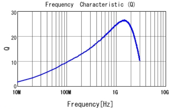
■ LQP03TN15NH02 Q
