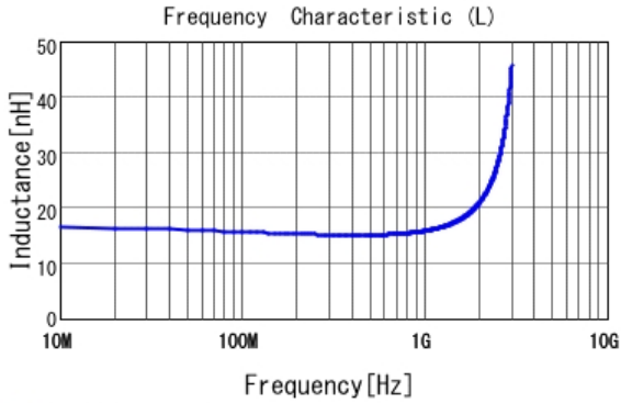
■ LQP03TN15NH02 L
