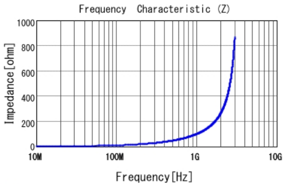
■ LQP03TN15NH02 |Z|
