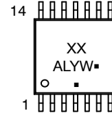
TSSOP-14 WB CASE 948G
