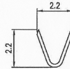
A-A SECTION
