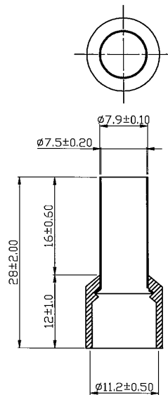
Dimensions : Millimetres
