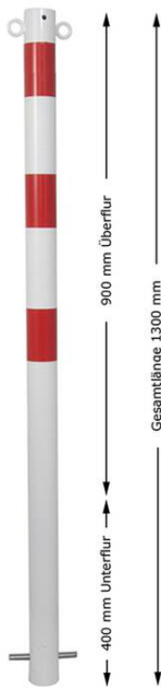
Modellbeispiel ortsfest zum Einbetonieren Art. 460b-2
