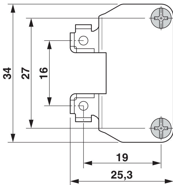
Maßzeichnung
