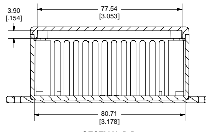
SECTION D-D
